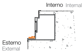
PORTA APERTA A 100° 100° OPEN DOOR
